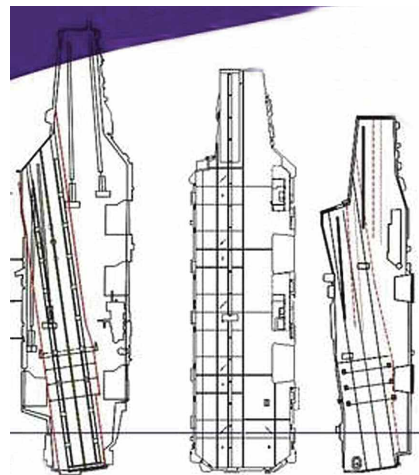
Aviācijas bāzes kuģu shematisks salīdzinājums. No kreisās: ASV «Nimitz» (ūdensizspāids — 91 t, 90 lidaparātu izvietošanas iespējas), Lielbritānijas CVF (65 t, 40 lidaparāti) un Francijas «Charles de Gaulle» (40 t, 40 lidaparāti).
