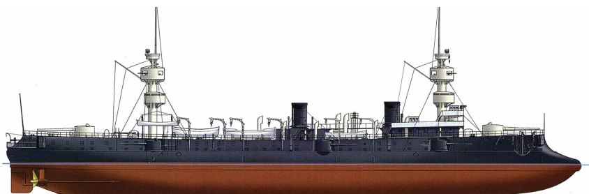
Bruņu kreiseris «Amiral Charner», Francija, 1894. gads. Ūdensizspāids — 4800 tonnas; izmēri — 137 x 14 x 6,3 metri; ātrums — 19 mezgli; apbruņojums — divi 193 mm un seši 138 mm lielgabali; bruņas (tērauda) — 92 mm bortiem, 110 mm torņiem, 40 mm klājam; apkalpe — 384—393 cilvēki.
