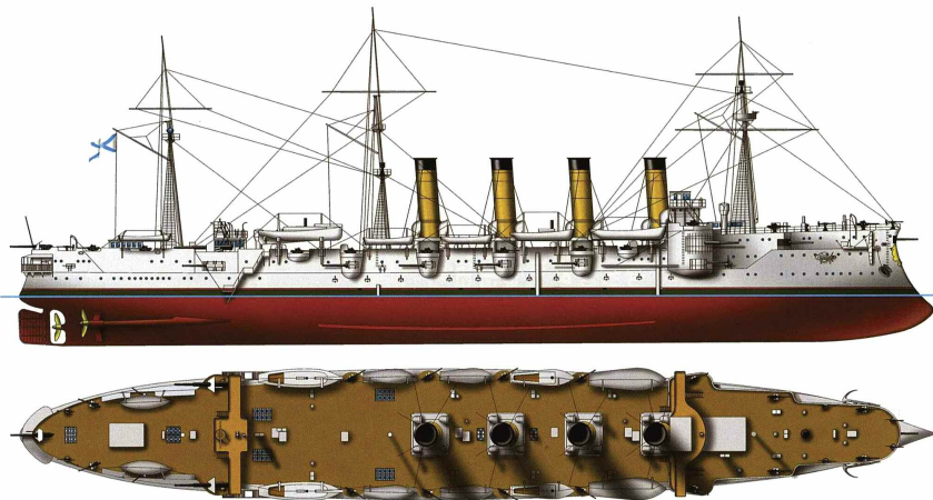
Bruņu kreiseris «Gromoboj», Krievija, 1900. gads. Ūdenssvars — 15 700 tonnas; izmēri — 146,6 x 20,88 x 8,48 metri; ātrums — 20 mezgli; apbruņojums — četri 203 mm un sešpadsmit 152 mm lielgabali; bruņas (tērauda) — 102—152 mm bortiem, 51—127 mm kazemātiem, 51—63 mm klājam; apkalpe — 814—877 cilvēki.
