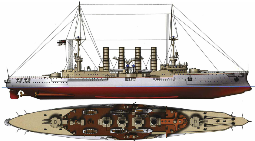
Bruņu kreiseris «Scharnhorst», Vācija, 1906. gads. Ūdensizspazids — 12 780 tonnas; izmēri — 144,6 x 21,6 x 8,37 metri; ātrums — 23,5 mezgli; apbruņojums — astoņi 210 mm, seši 150 mm un astoņpadsmit 88 mm lielgabali; bruņas (tērauda) — 100—150 mm bortiem, 120—150 mm kazemātiem, 170 mm torņiem, 35+55 mm klājiem; apkalpe — 764 cilvēki.
