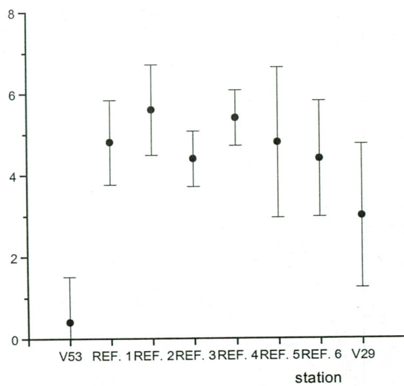
Fig. 6: Vissen op Loswal Noord en referentiestations Gemiddeld aantal soorten per schaaftrek + 95% betrouwbaarheidsgrenzen.
