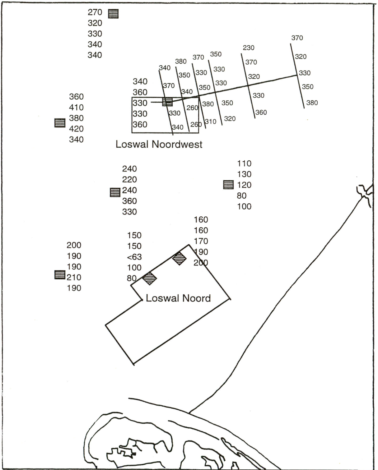
Fig. 4: Mediane korrelgrootte (µm) van het sediment (inclusief de slibfractie) op en rond Loswal Noord en Loswal Noordwest.
