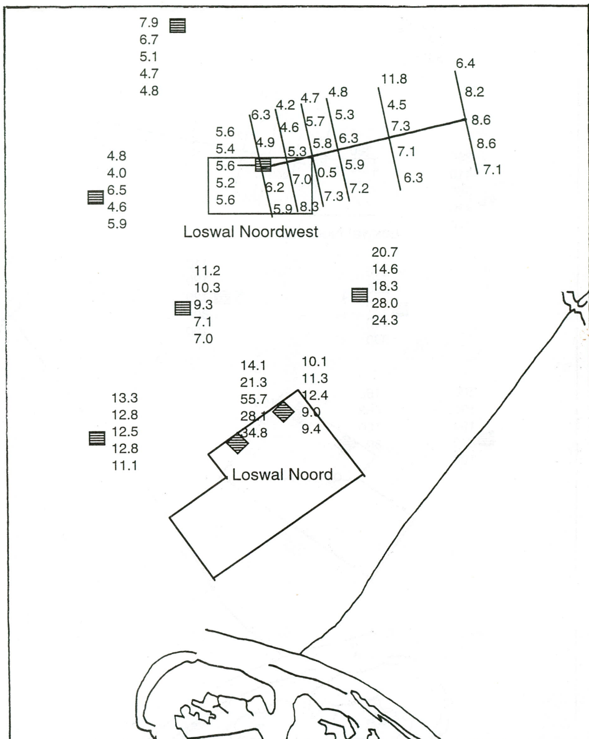
Fig. 3: Slibgehalten (totale fraktie < 16 \mu\text{m} , %) van het sediment op en rond Loswal Noord en Loswal Noordwest.
