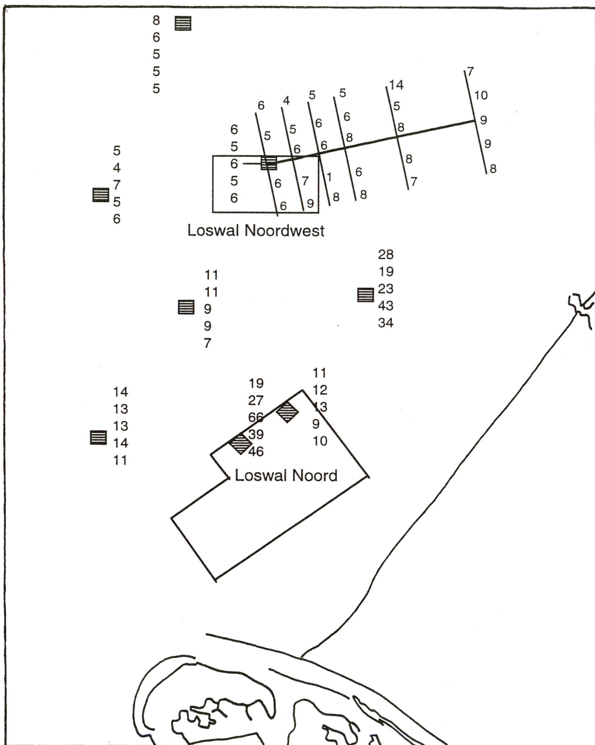
Fig. 2: Slibgehalten (totale fraktie <math><63 \mu\text{m}</math>, %) van het sediment op en rond Loswal Noord en Loswal Noordwest.
