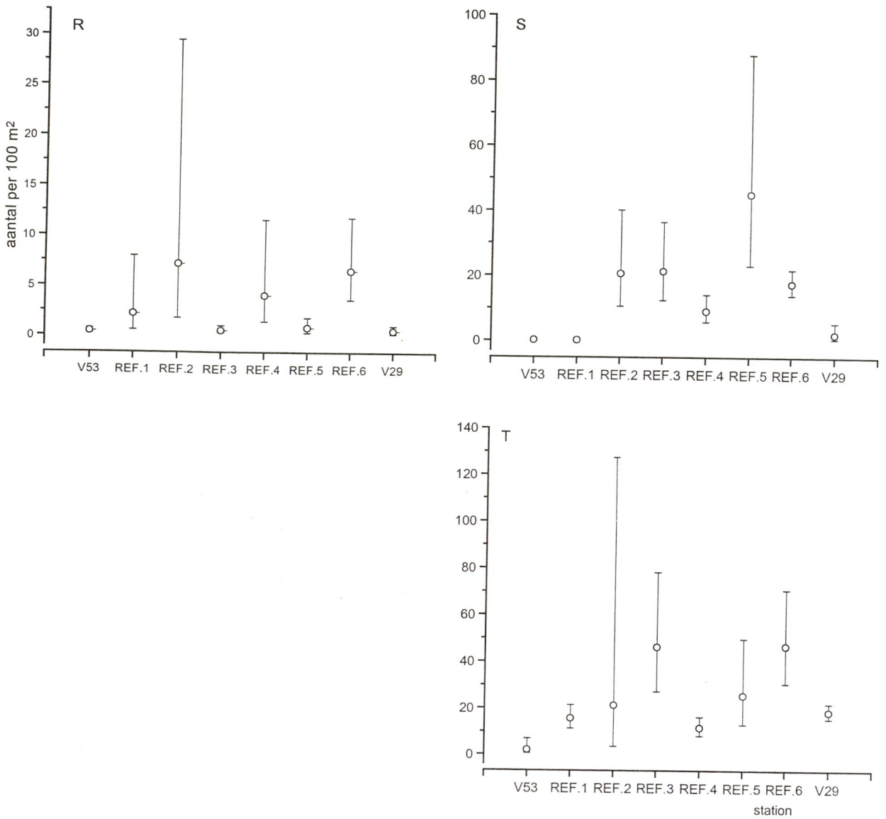
Fig. 10R-T: Gemiddelde dichtheden van 3 soorten kreeftachtigen (Crustacea) op Loswal Noord en de referentiestationen. De 95% betrouwbaarheidsgrenzen zijn aangegeven.
