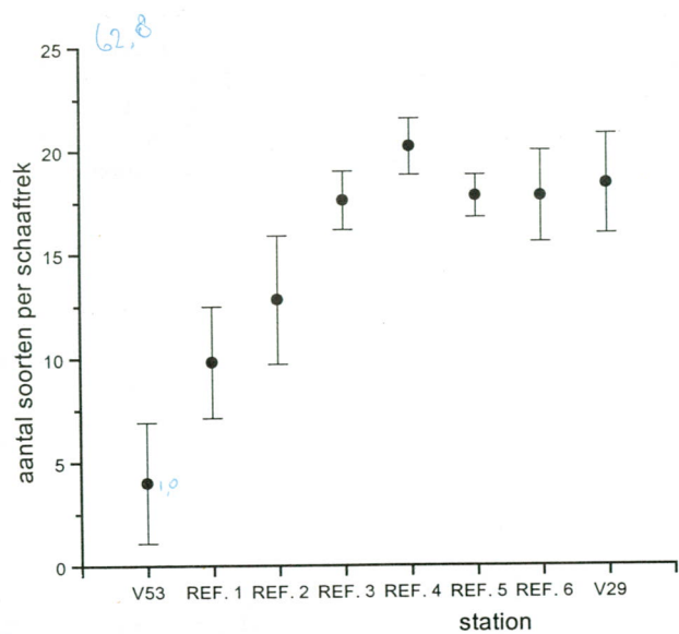
Fig. 5.: Makrobenthos Loswal Noord en referentiestations Gemiddeld aantal soorten per schaaftrek + 95% betrouwbaarheidsgrenzen.
