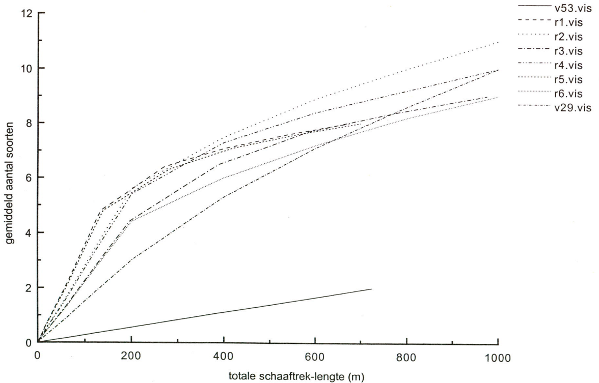
Fig. 7: Rarefaction curves voor makrobenthos (boven) en vissen (onder). Per station is het gemiddeld aantal soorten uitgezet dat is aangetroffen nadat een toenemend aantal schaaftrekken is uitgevoerd, resp. een toenemend aantal meters bodem met de schAAF is bemonsterd.
